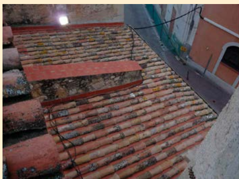
Imatge general de la coberta per on es produeixen filtracions d'aigua.
